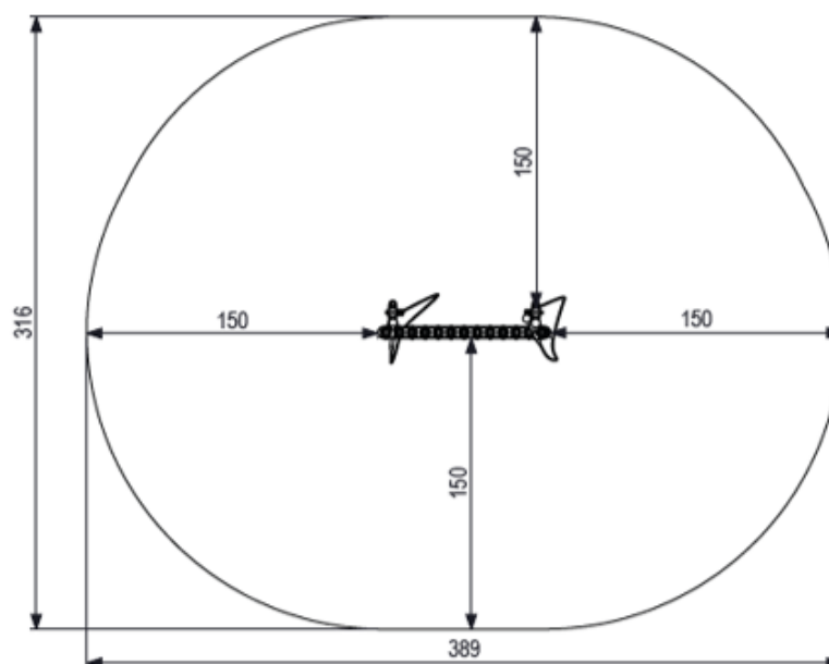
Voetenplan SCALE 1:8
