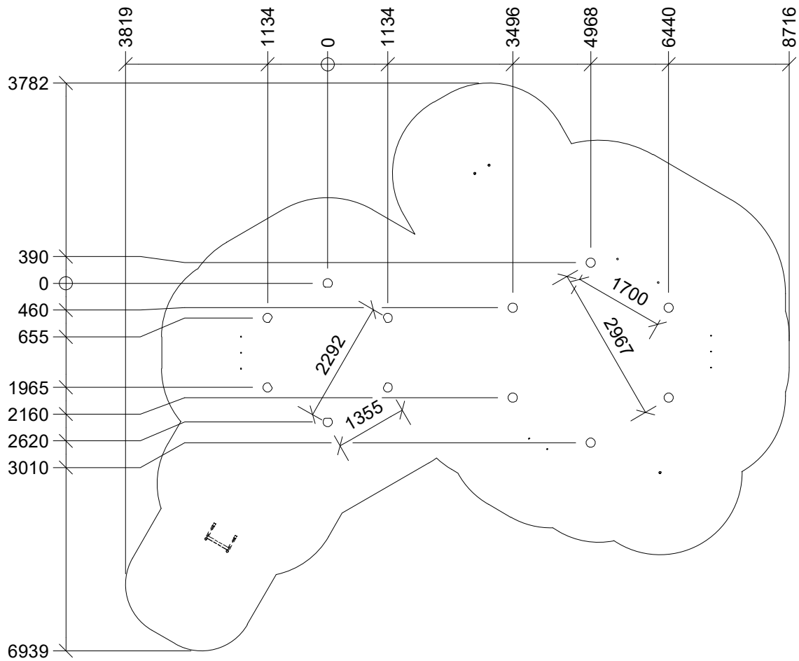
A-A ( 1 : 100 )
