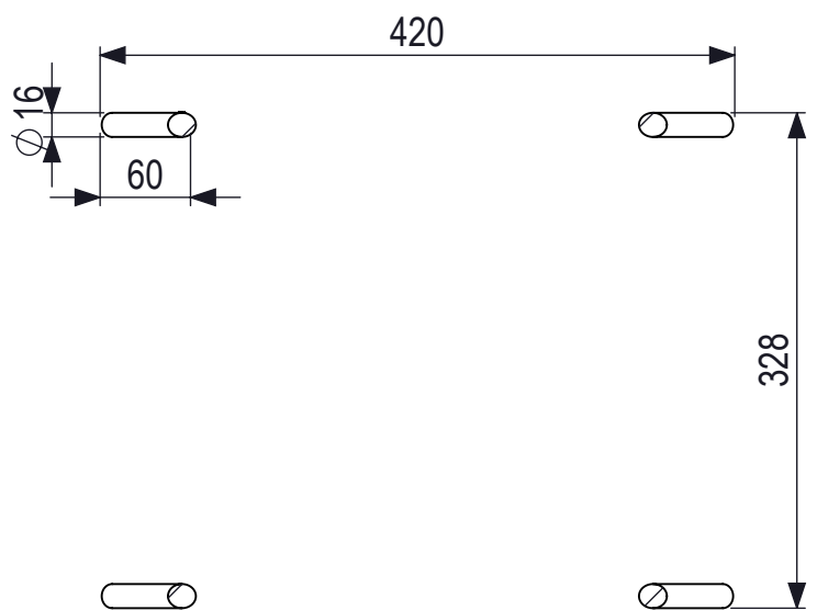
Voetenplan
