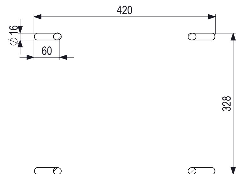
Voetenplan
