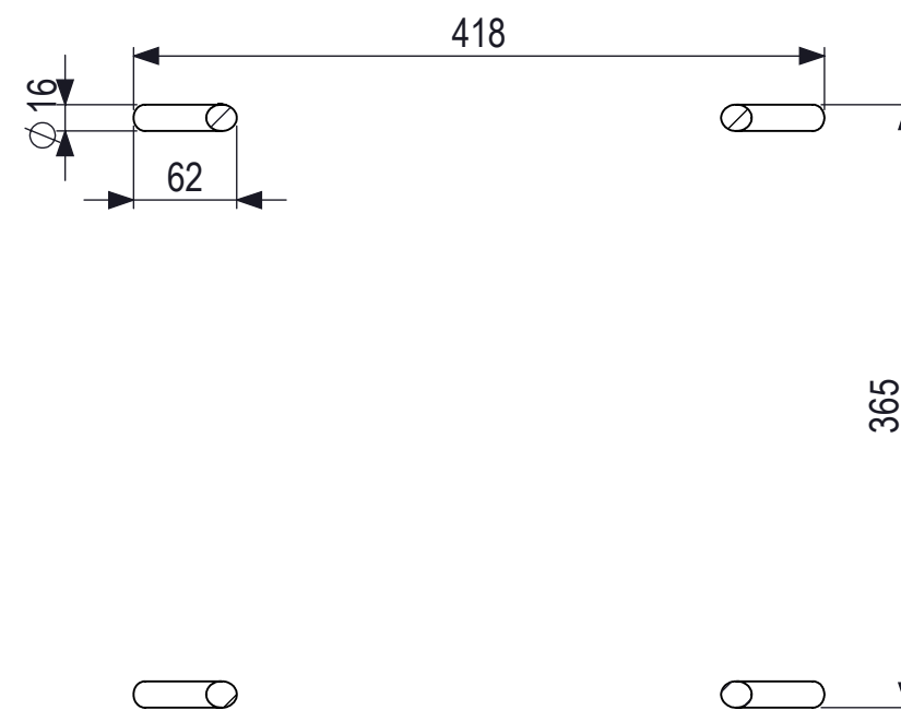
Voetenplan
