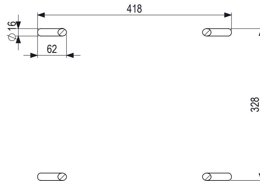
Voetenplan
