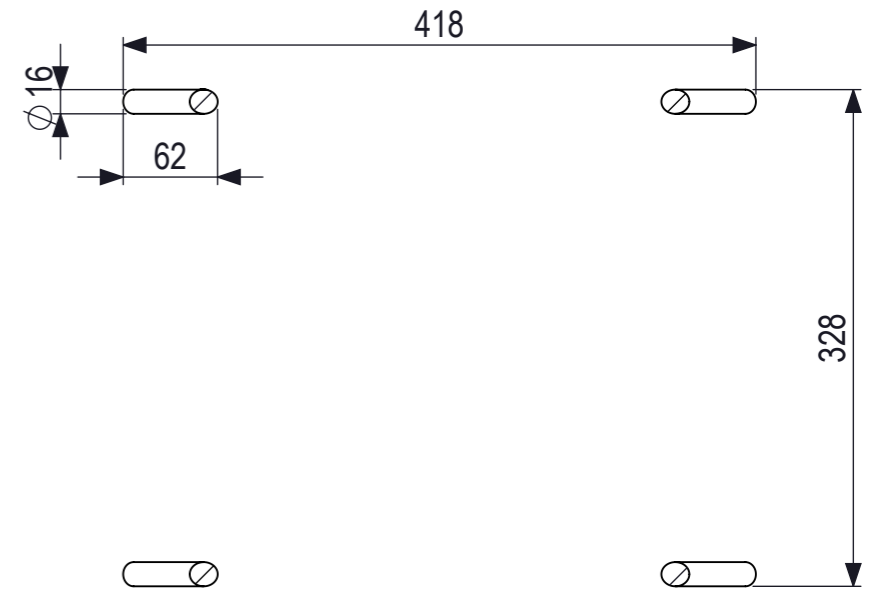
Voetenplan
