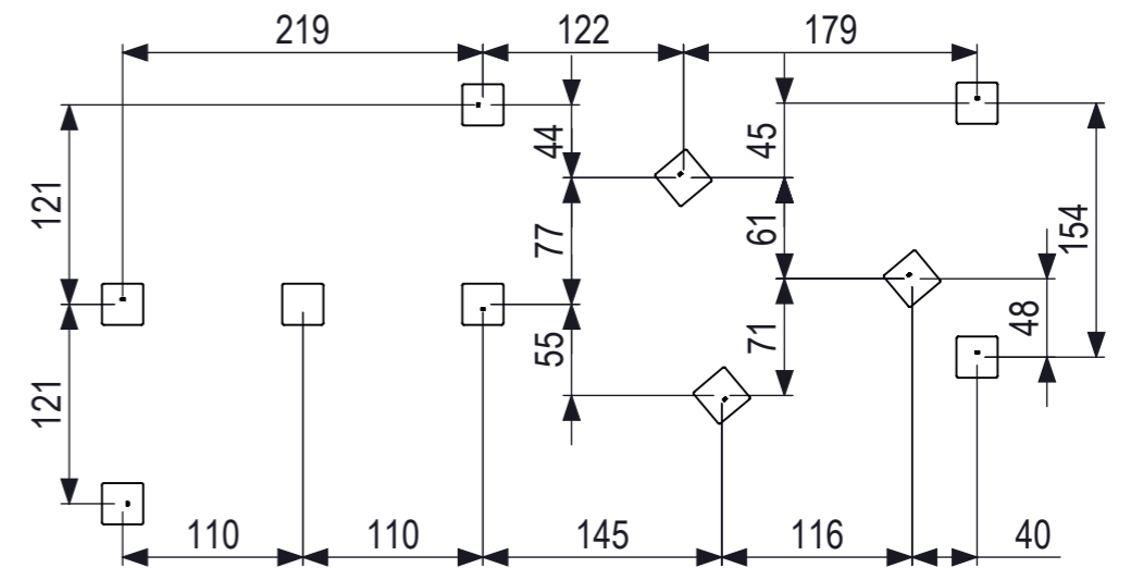
Fundatieplan SCALE 1:50
