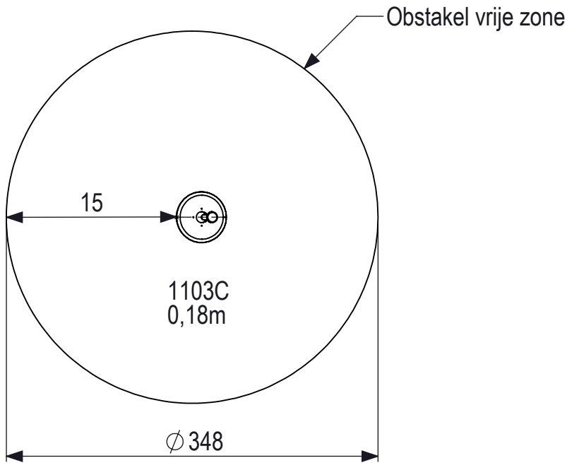
Bovenaanzicht schaal 1:50
