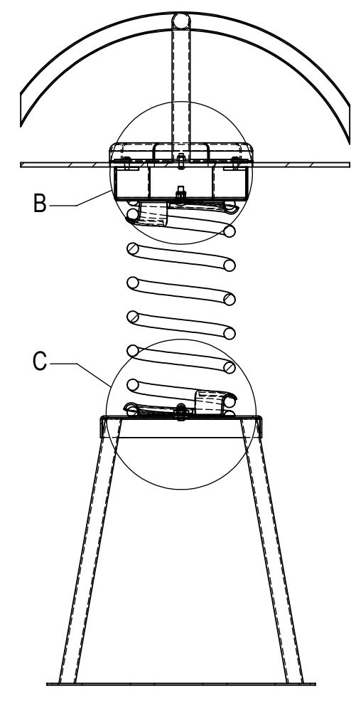
SECTION A-A
