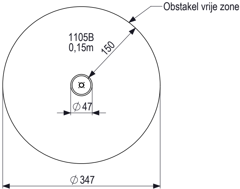
Bovenaanzicht schaal 1:50
