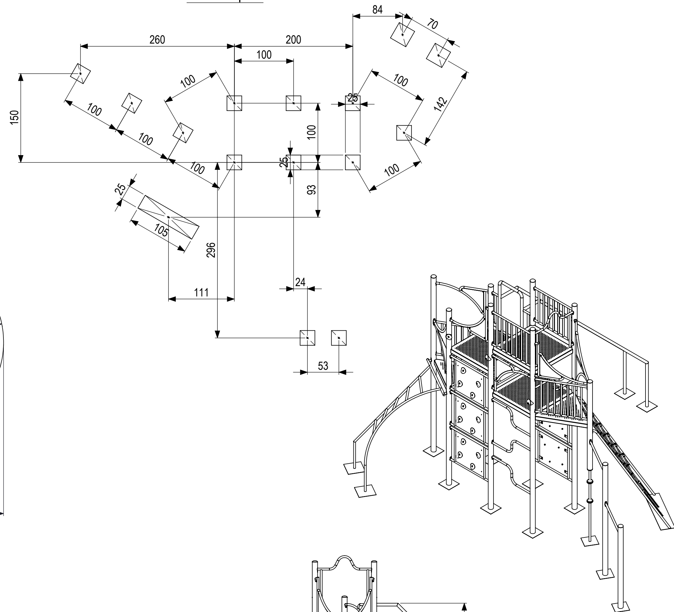
Fundatieplan
